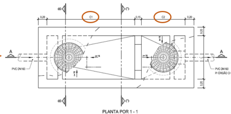
PLANTA POR 1 - 1
