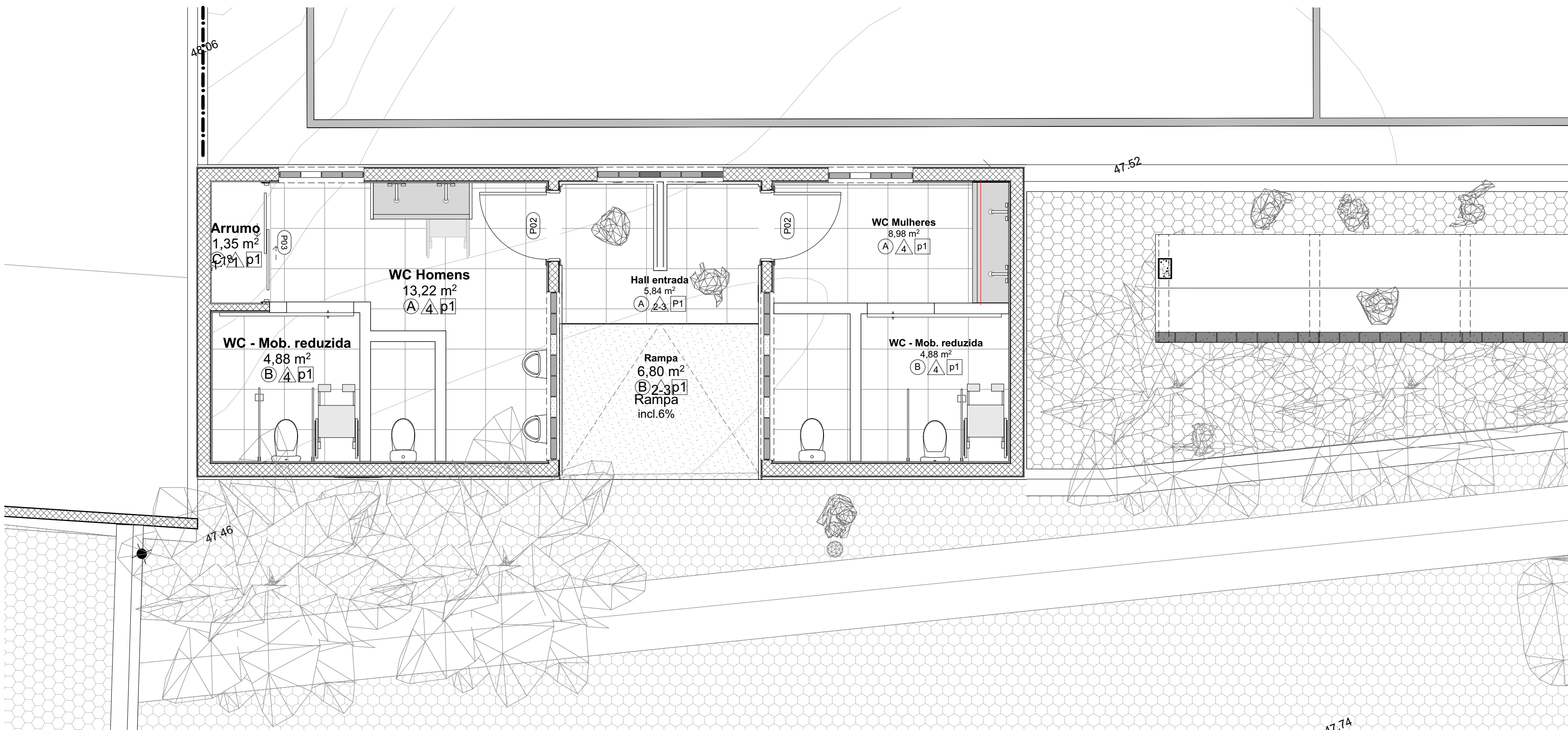
P9B_SC_R_CHB-ARQ-120-07 PLANTA DE ACABAMENTOS Escala: 1:50
