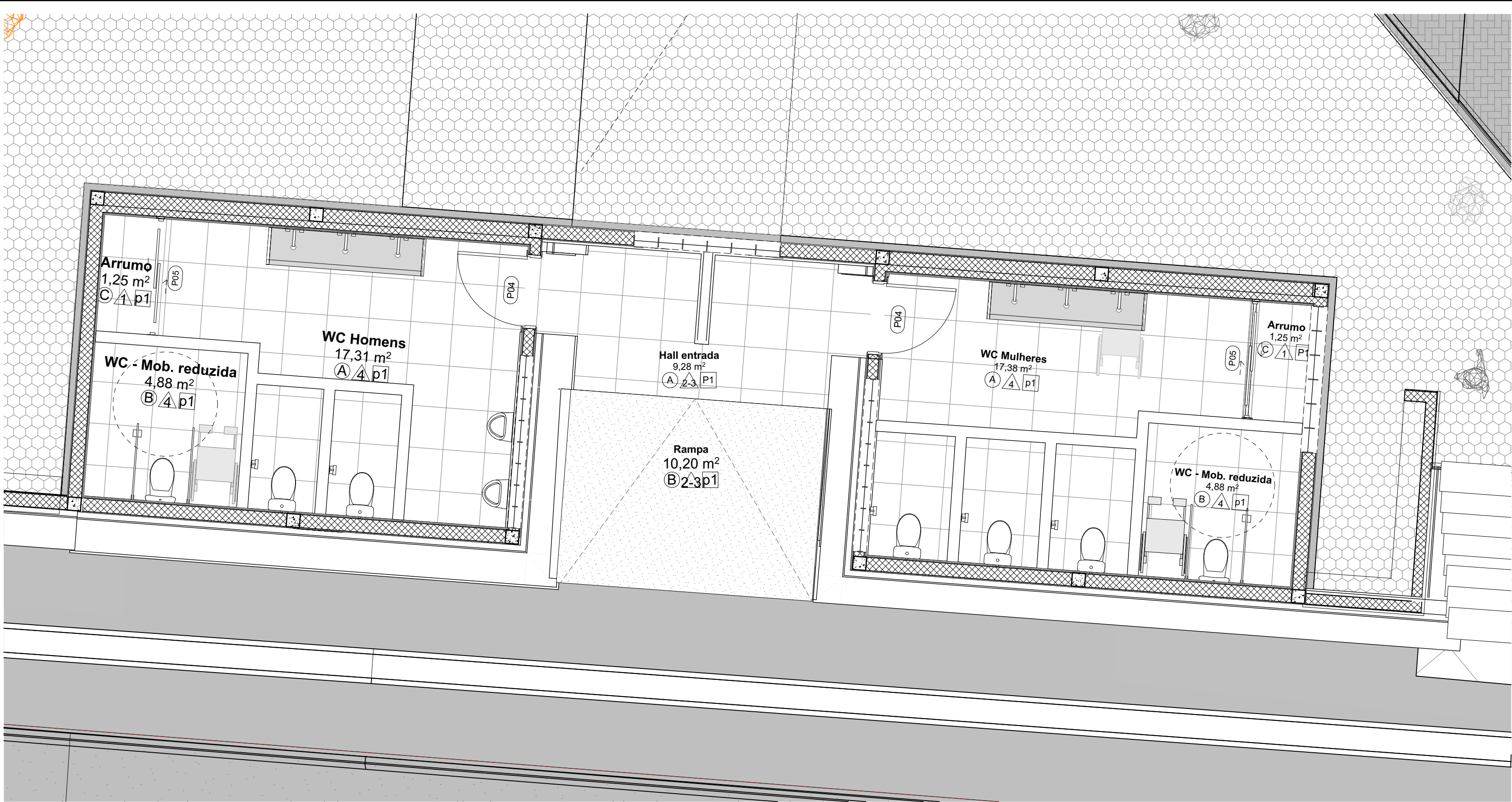
P9B_SC_RE_ML-ARQ-120-08 PLANTA DE ACABAMENTOS Escala: 1:50
