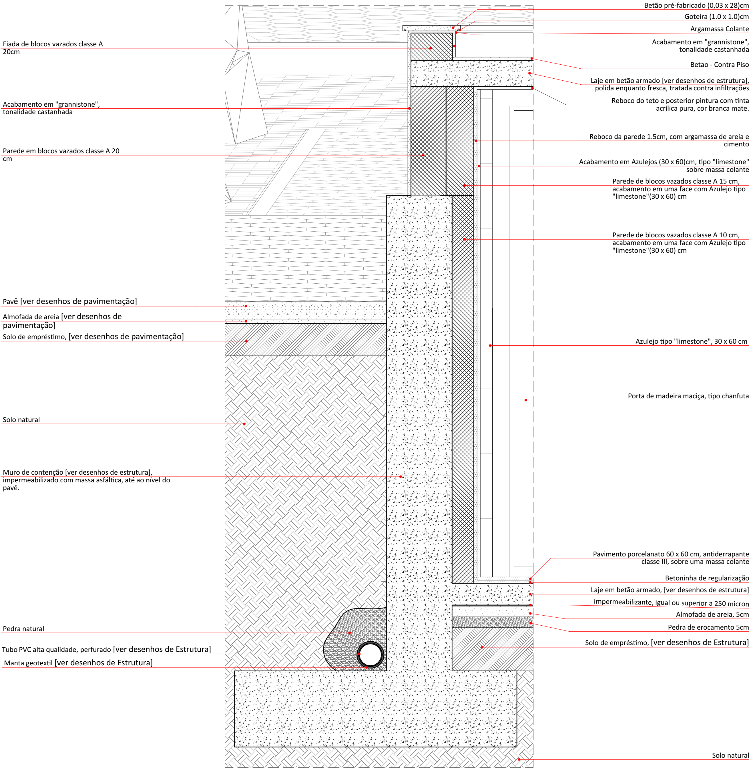
P9B_SC_PO_ML-ARQ-130-03 D-01 Det. Escala: 1:10
