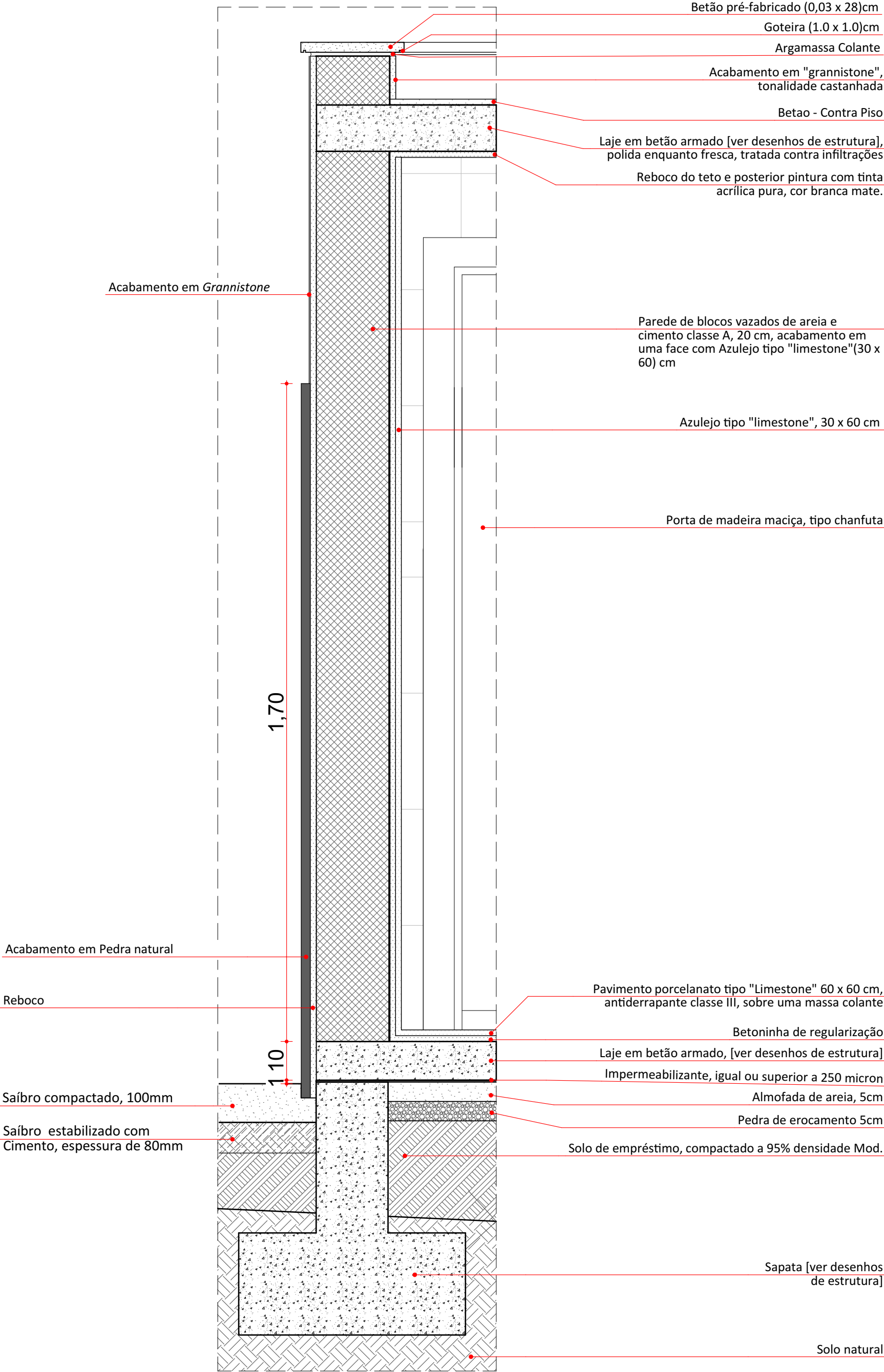
P9B_SC_PC_CHB-ARQ-130-04 PORMENOR DE CONSTRUÇÃO Escala: 1:10
