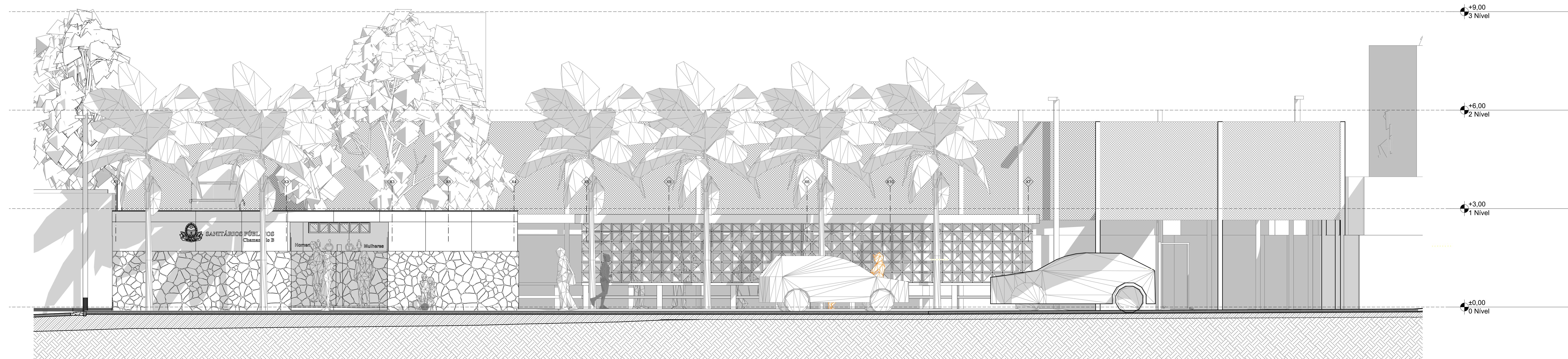
P9B_SC_EL_CHB-ARQ-130-07 Elevação 1 Escala: 1:50
