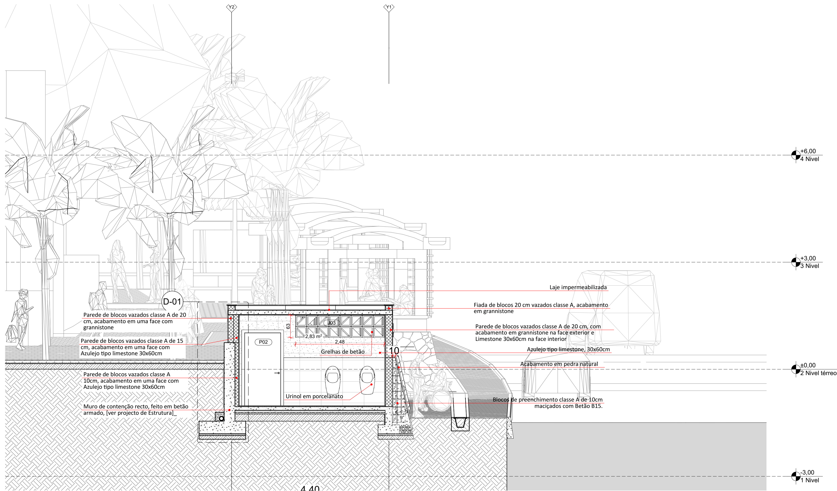
02 CORTE - D-WC Escala: 1:50
