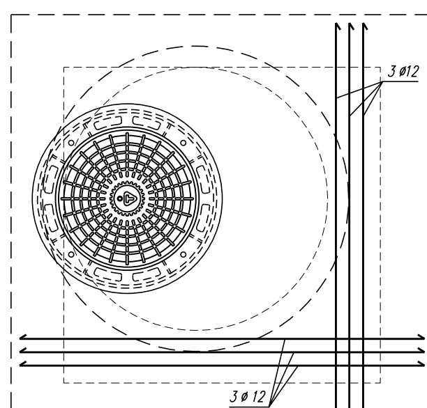
PLANTA (ARMADURA EM AMBAS AS FACES)
