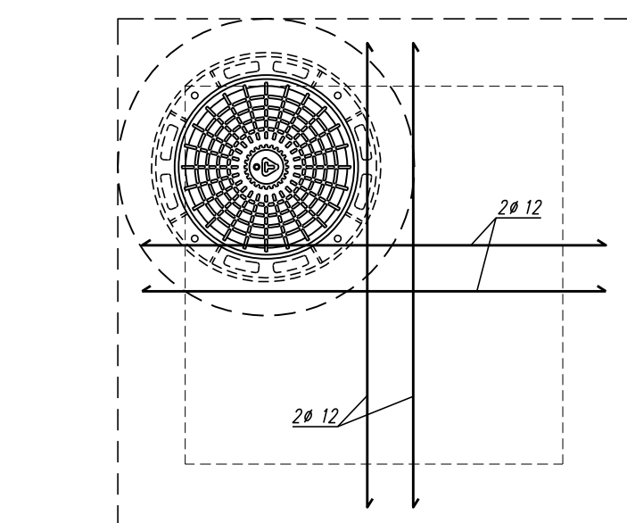
PLANTA (ARMADURA EM AMBAS AS FACES)
