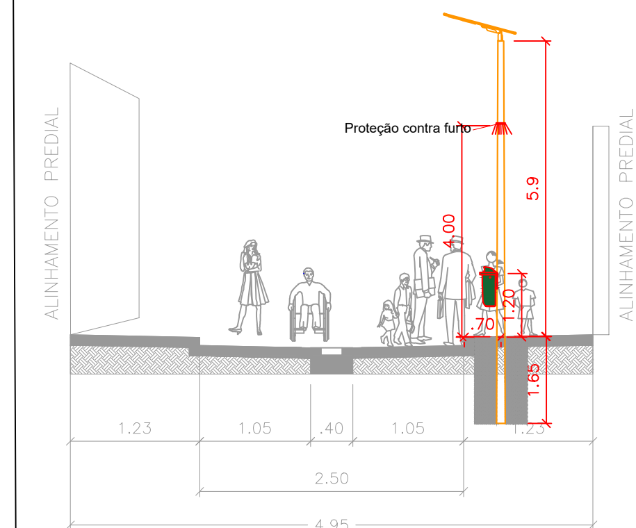
VIAS DE MOB.COMPART. E ACESSIBILIDADE ESCALA 1:50
