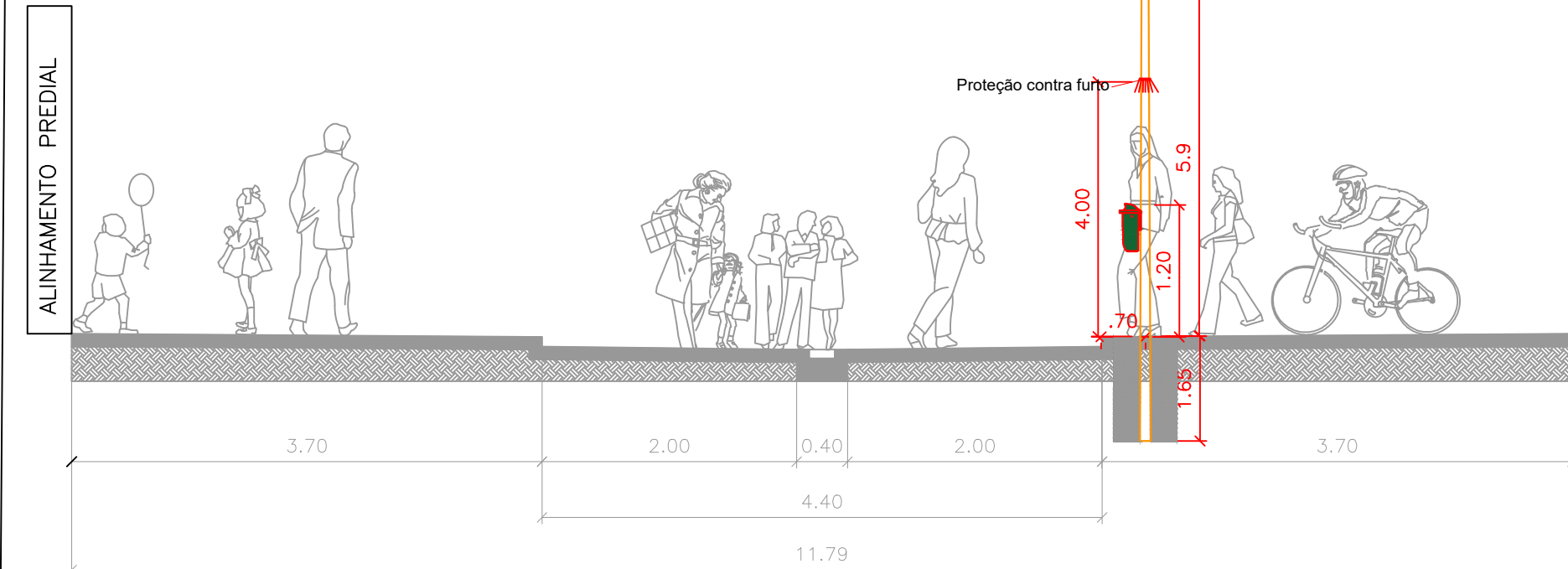
CORTE C - C VIAS DE MOBILIDADE COMPARTILHADA ESCALA 1:50
