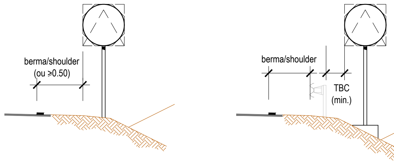
SEM GUARDA METÁLICA/NO GUARDRAIL
