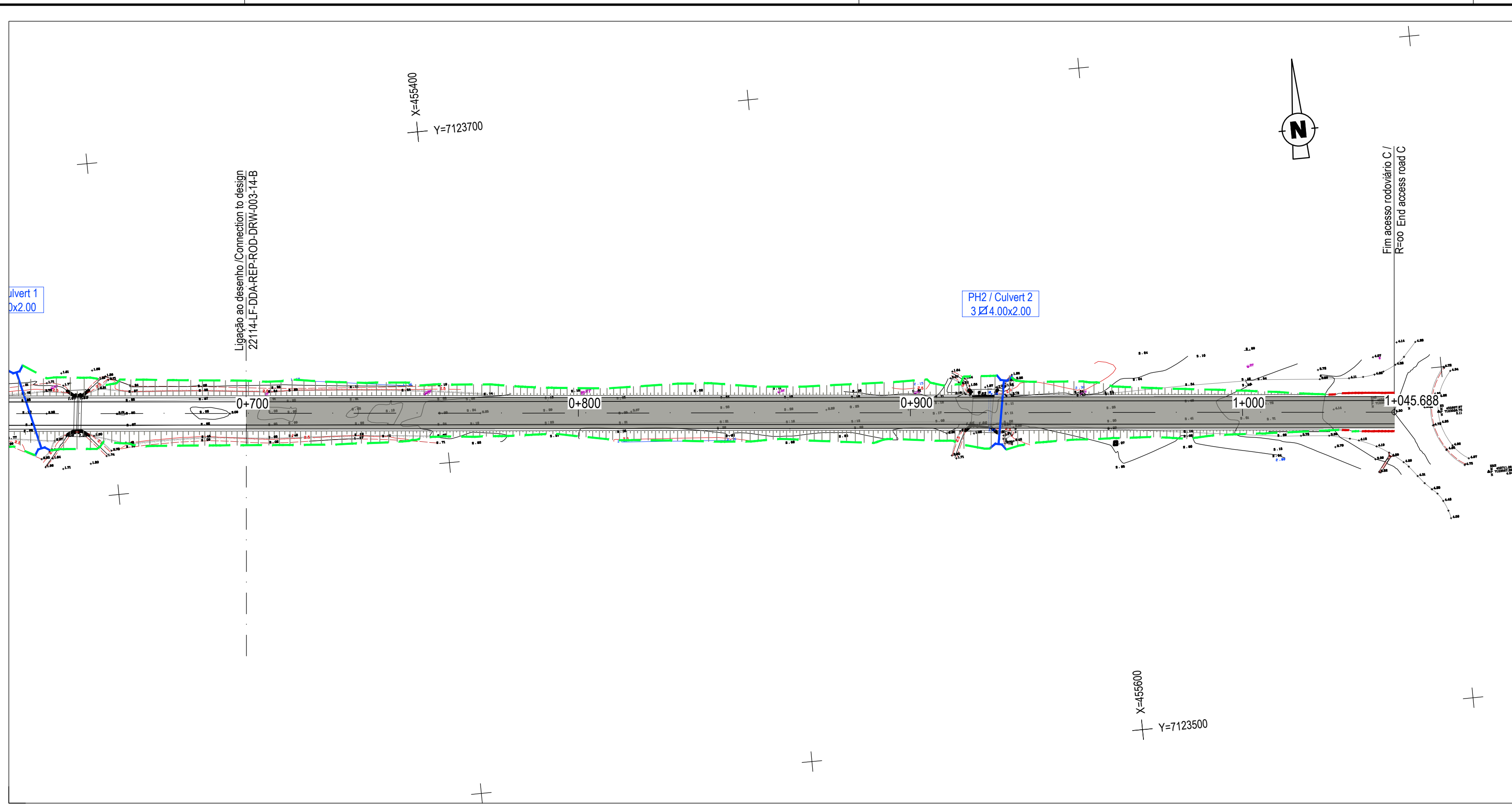
ACESSO RODOVIÁRIO C / ACCESS C ROAD PLANTA / PLAN Escala / Scale 1:1000
