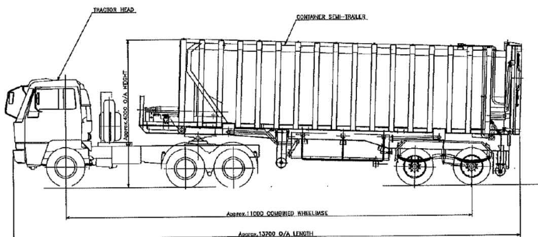
Figura 4-8 Camiões semi-reboque de transporte de RSU
