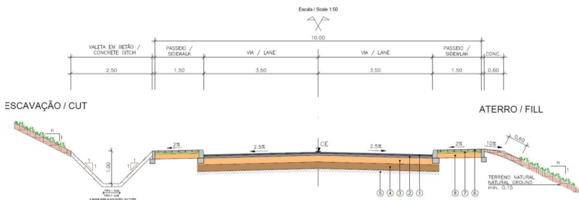
Figura 4-6 Perfil transversal tipo (secção corrente).
