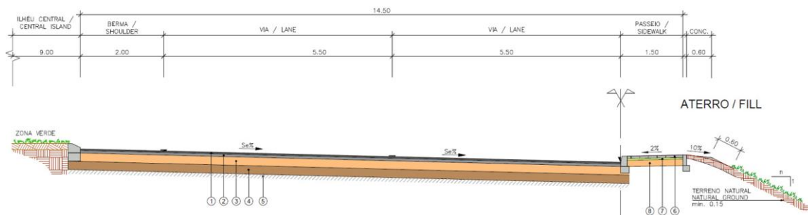
Figura 4-7 Perfil transversal tipo (rotundas).
