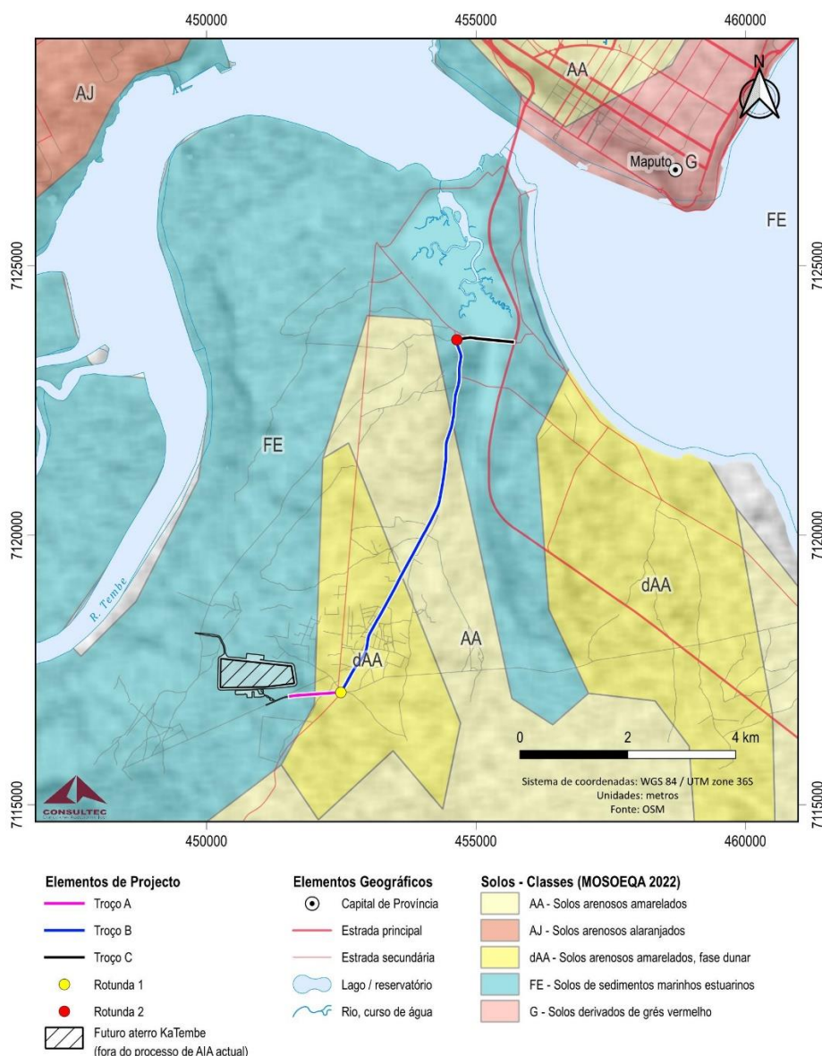
Figura 6-19 Unidades de Solos presentes na área em estudo
