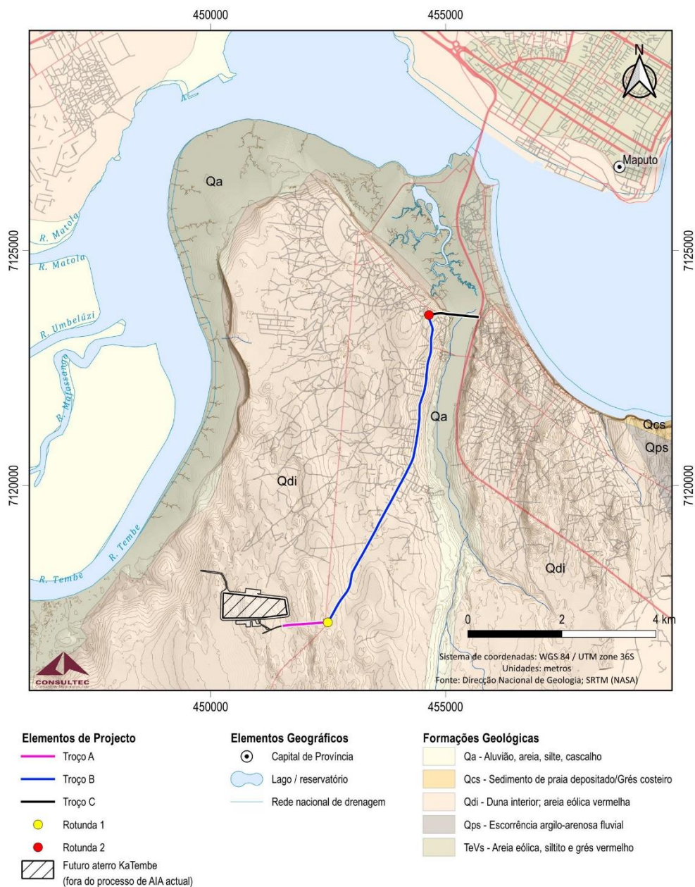
Figura 6-18 Formações geológicas presentes na área do Projecto
