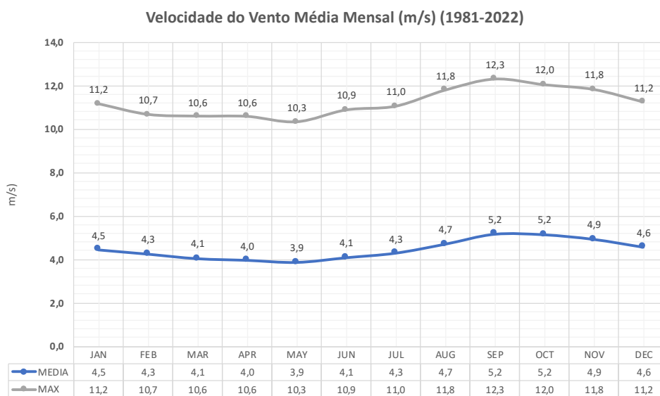
Figura 6.4 – Velocidade do vento média mensal
