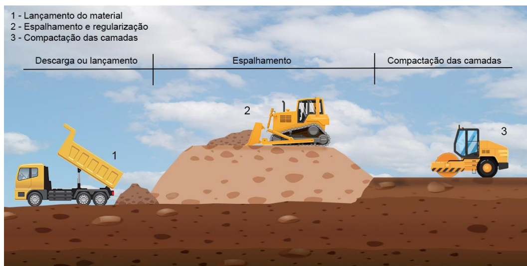
Figura 4-11 Etapas de construção de aterros
